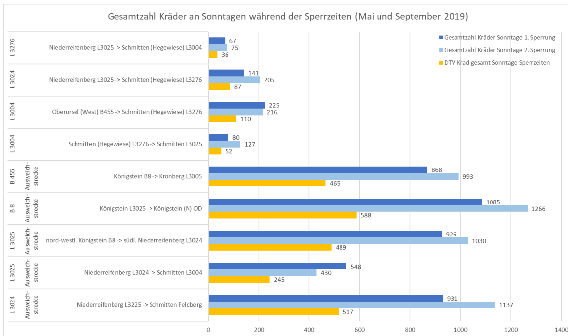
Abb 3: Verkehrsaufkommen Motorräder gesamt (absolut) und DTV an den Sonntagen mit Sperrung im Mai und September 2019
