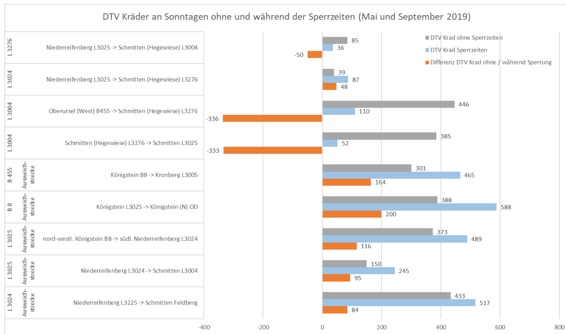
Abb. A 7: Diagramm - Veränderung Motorradverkehrsaufkommen (DTV) an Sonntagen mit und ohne Sperrung
