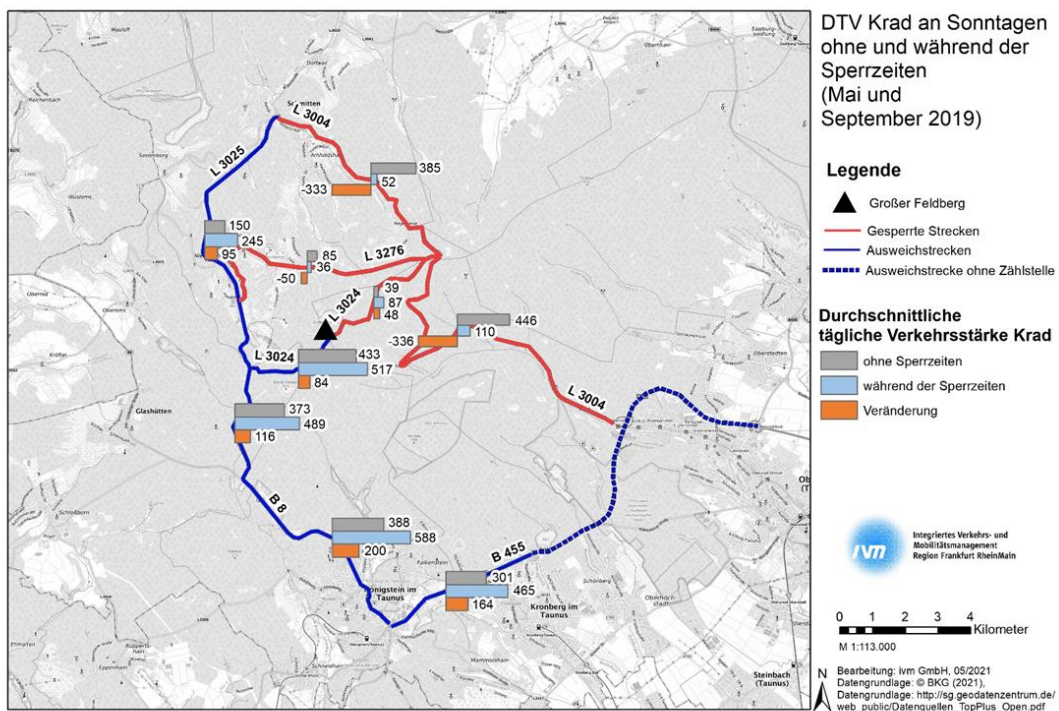
Abb. A6: Veränderung des DTV Krad an Sonntagen mit und ohne Sperrung
